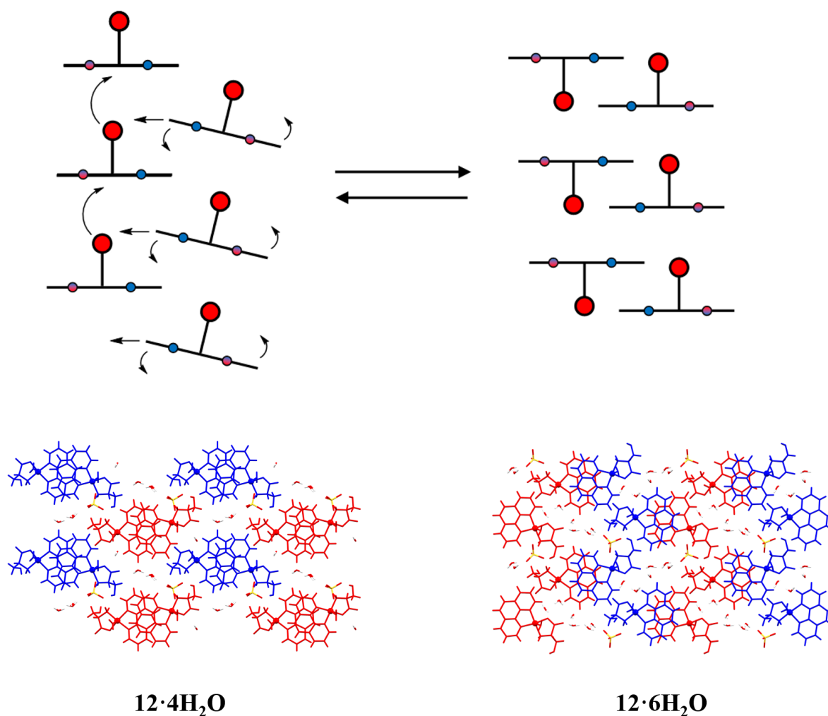
Slika 98. Shematski prikaz mogućeg mehanizma pomaka atoma tijekom transformacije jednog solvata u drugi. Dan je primjer transformacije 12a \cdot 4H_2O \rightleftharpoons 12a \cdot 6H_2O . Na donjim slikama su prikazi pakiranja molekula u kristalu u ravninama okomitim na prostiranje dvostrukih lanaca. Crvenom bojom su označeni kompleksi usmjereni na način \uparrow , a plavom bojom kompleksi usmjereni na način \downarrow .
