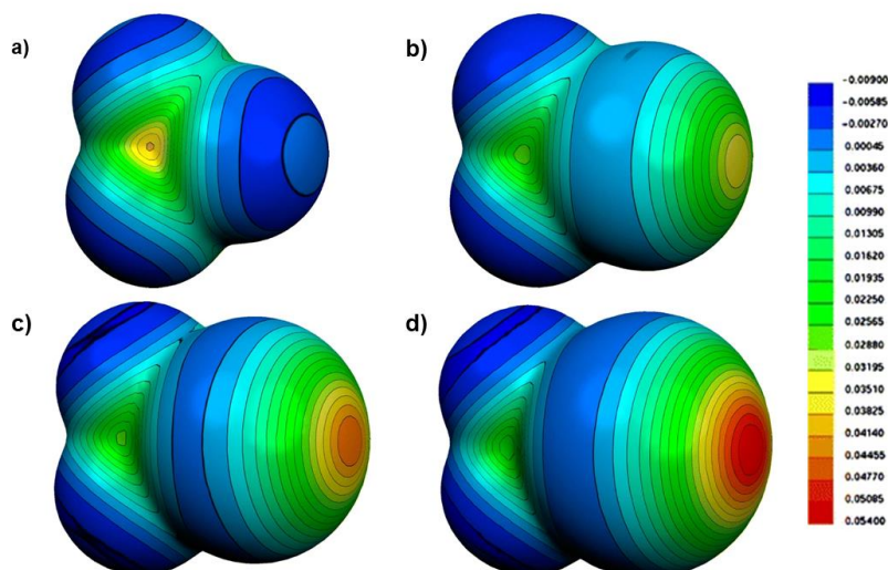
Slika 3. Elektrostatski potencijal (ESP) na izoplohi elektronske gustoće a) tetrafluormetana b) trifluorklormetana c) bromtrifluormetana d) trifluorjodmetana u Hartreeima pri rezoluciji 0,001 Bohr -3 . Preuzeto s ref. 21
