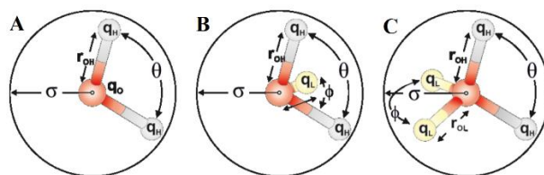
Slika 4. A) Modeli s 3 točkasta naboja koji uključuju SPC i TIP3P, B) model s 4 točkasta naboja kao TIP4P i C) model s 5 točkastih naboja poput TIP5P. Slika preuzeta iz 2 .
