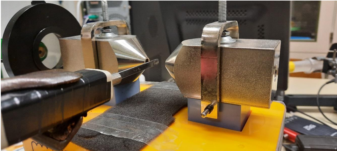
Slika 9. Hallova sonda između magneta. Vrh Hallove sonde nalazi se na pravcu koji spaja rupe elektro-magneta te se svako mjerenje pomiče od lijeva ka desno za zadanu udaljenost. Udaljenost i broj točaka ovisi o uzorku za koji se mjeri magnetsko polje.
