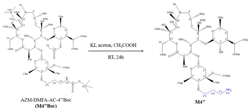
Slika 39. Reakcijska shema dobivanja produkta M4'' .
