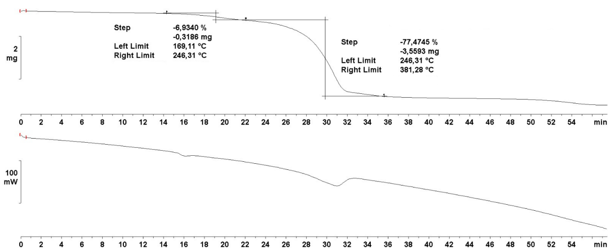
Slika D27. TG i DSC krivulje R\text{-(DAP)}_4\text{CuCl}_{10}
