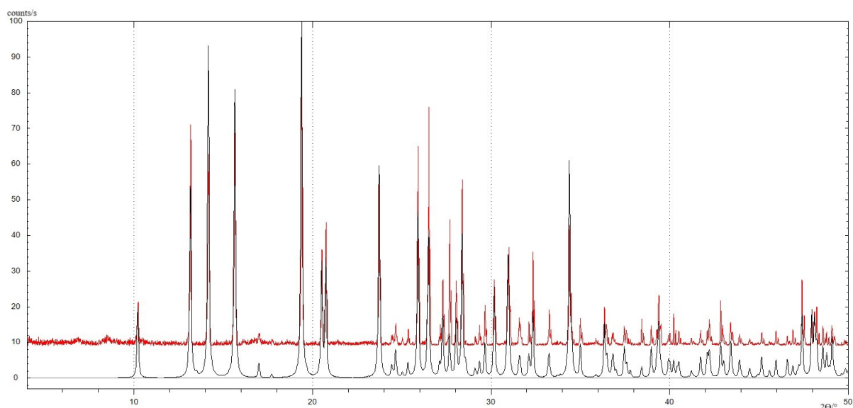
Slika D6. Usporedba difraktograma prahe R -(DAP)[ZnCl 4 ]·H 2 O priređenog otopinskom sintezom (crveno) i simuliranog difraktograma prahe R -(DAP)[ZnCl 4 ]·H 2 O izračunatog na temelju podataka difrakcije rendgenskih zraka na jediničnom kristalu (crno)
