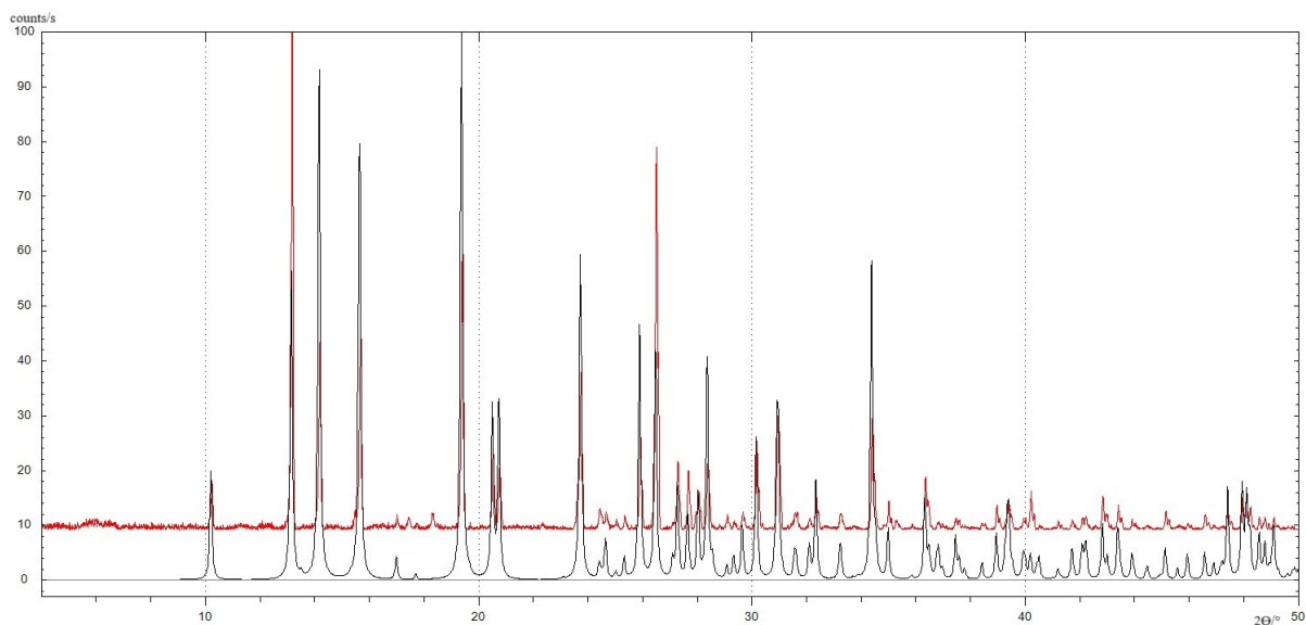
Slika D5. Usporedba difraktograma prahe rac -(DAP)[ZnCl 4 ]·H 2 O priređenog otopinskom sintezom (crveno) i simuliranog difraktograma prahe rac -(DAP)[ZnCl 4 ]·H 2 O izračunatog na temelju podataka difrakcije rendgenskih zraka na jediničnom kristalu (crno)
