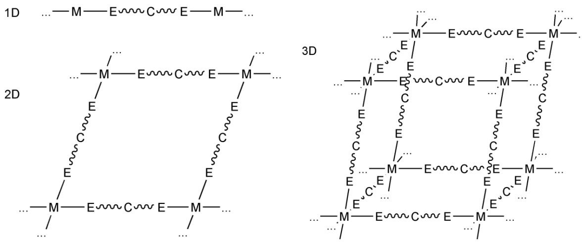
Slika 1. Shematski prikaz 1D, 2D i 3D koordinacijskog polimera. M označava atom metala, a E-C-E organski premosni ligand.
