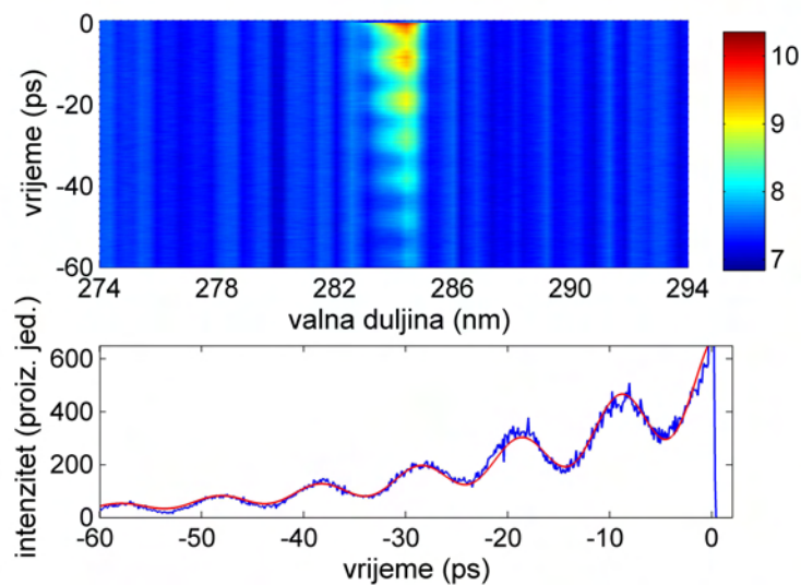
Slika 5.15: Kvantni udari na 285\ \text{nm} perioda 9.8\ \text{ps} zbog trofotonskog pobuđenja 5p nivoa pulsevima podešenima na \lambda_c = 854\ \text{nm} snimljeni spektrometrom. Donji dio slike prikazuje tranzijent na valnoj duljini od 285\ \text{nm} te prilagodbu na izraz 5.3.9. p(\text{He})=25\ \text{Torr} , T_{\text{Na}} = 425^\circ\text{C} ( N_{\text{Na}} = 9.9 \times 10^{15}\text{cm}^{-3} ). P_{\text{ulaz}} = 2\ \mu\text{J} . Pri većim snagama titraji nestaju.
