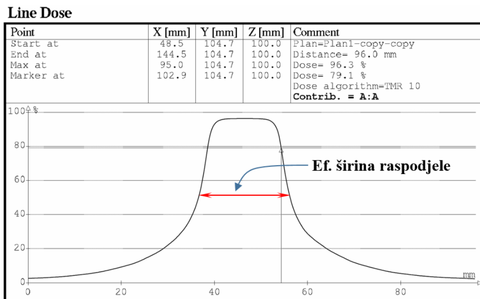
Slika 2.32 Primjer simuliranog LL-profila doze za 18 mm-sku kolimatorsku kacigu. Izvan efektivne širine raspodjele 2R^k profil opada bitno sporije nego unutar raspodjele.
