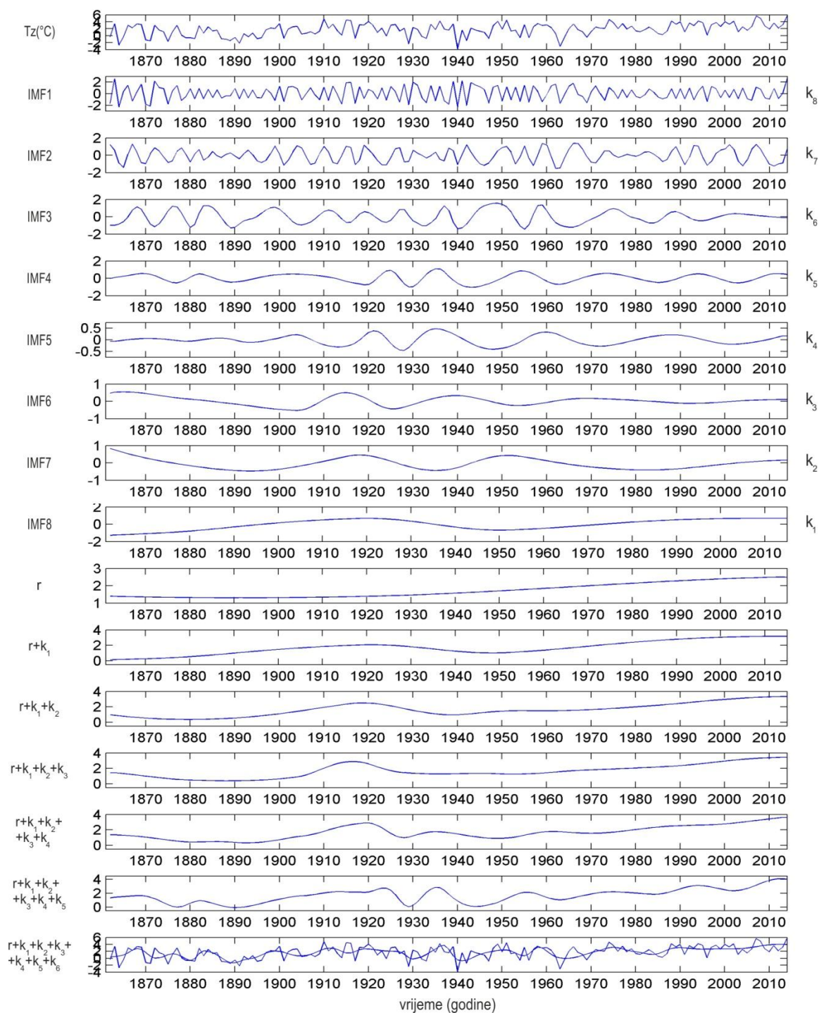
Slika D1. Vremenski niz zimskih srednjaka temperature, IMF dobivene primjenom EMD metode na taj niz, reziduom r te kumulativne sume reziduuma i odgovarajućih komponenti ( r+k_1 , r+k_1+k_2 ...)
