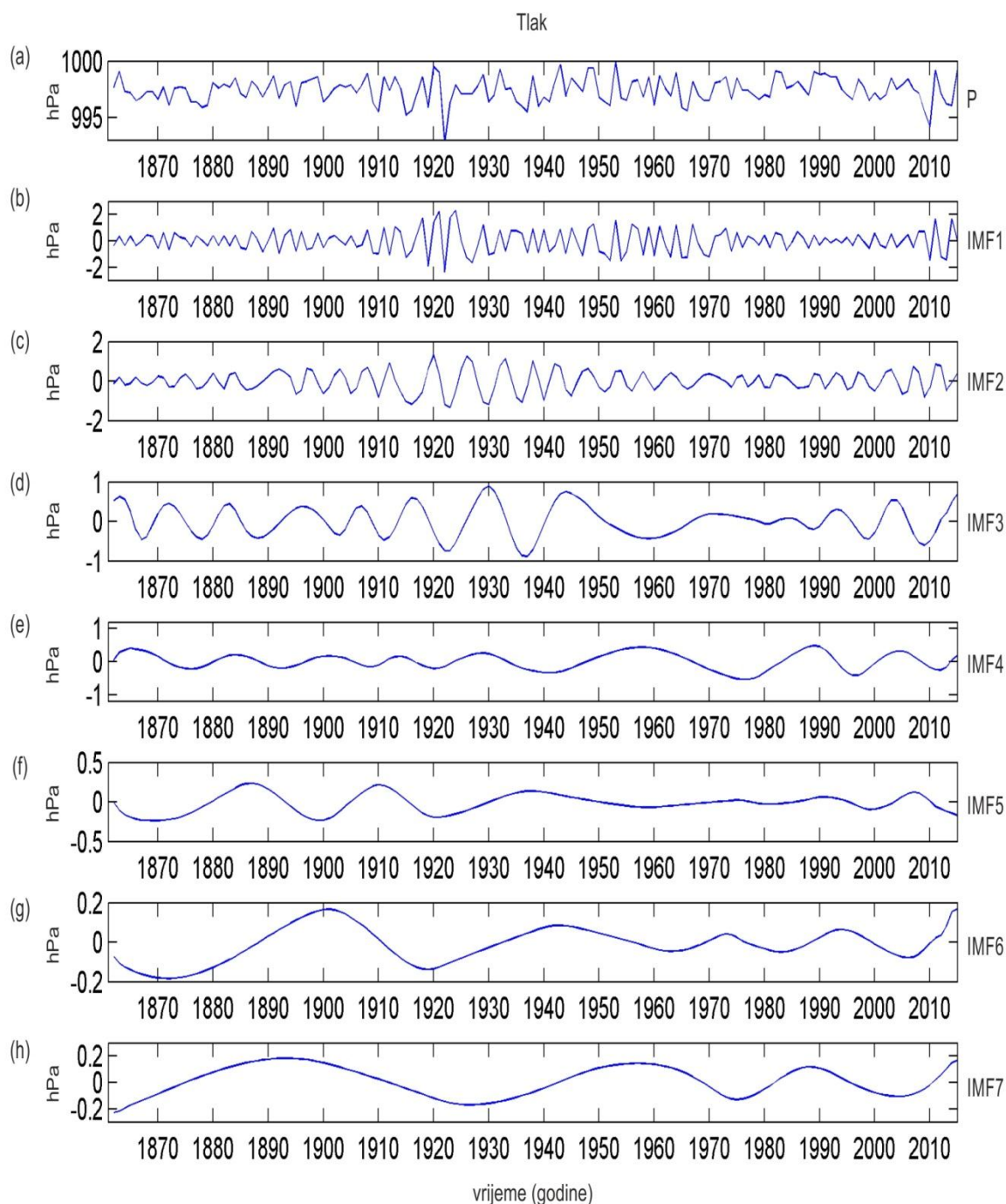
Slika 8. Isto kao slika 2, samo za niz godišnjih srednjaka tlaka zraka.
