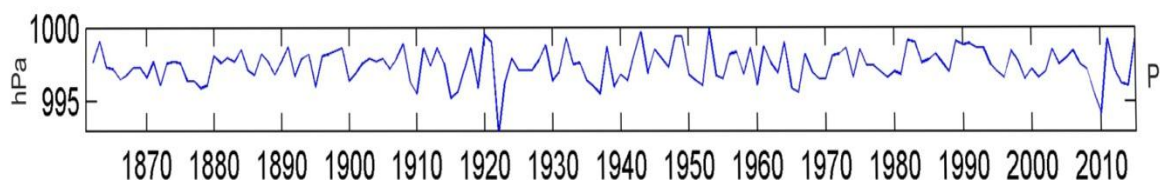
Slika 11. Niz godišnjih srednjaka tlaka zraka.
