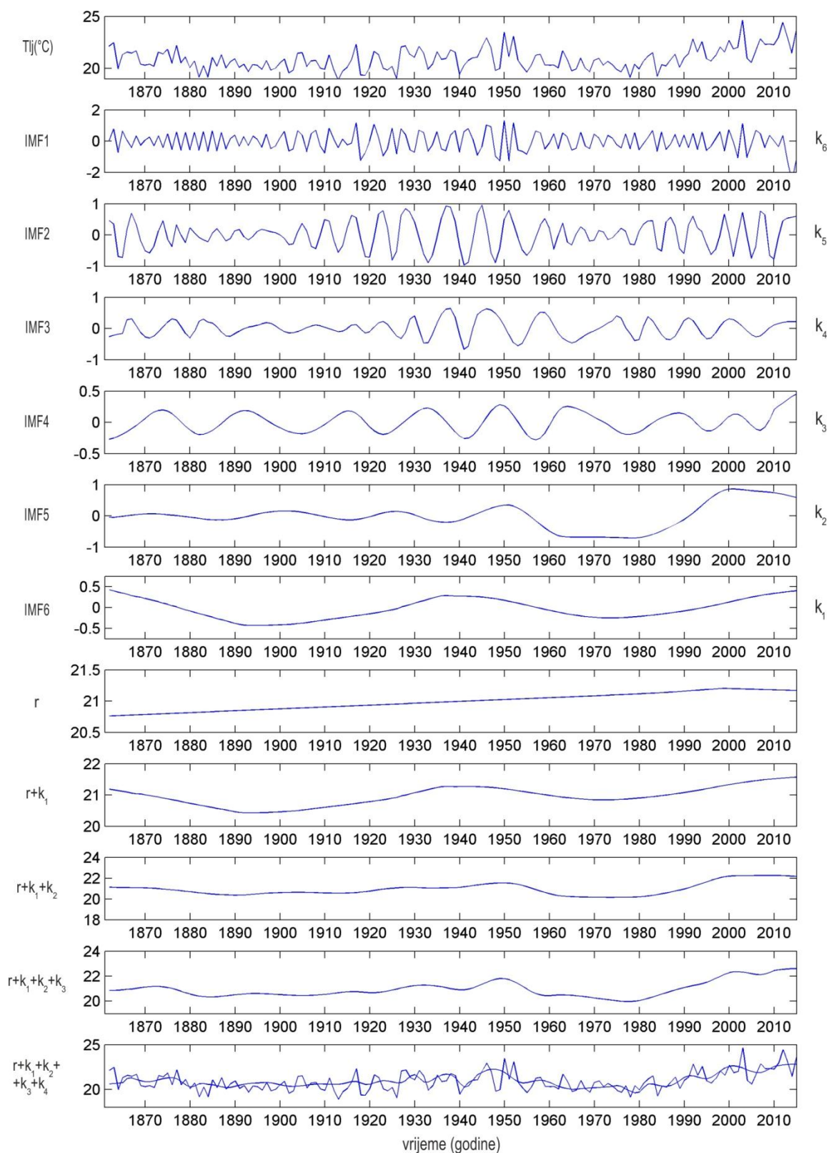
Slika D3. Isto kao slika D1 samo za ljetne temperature.
