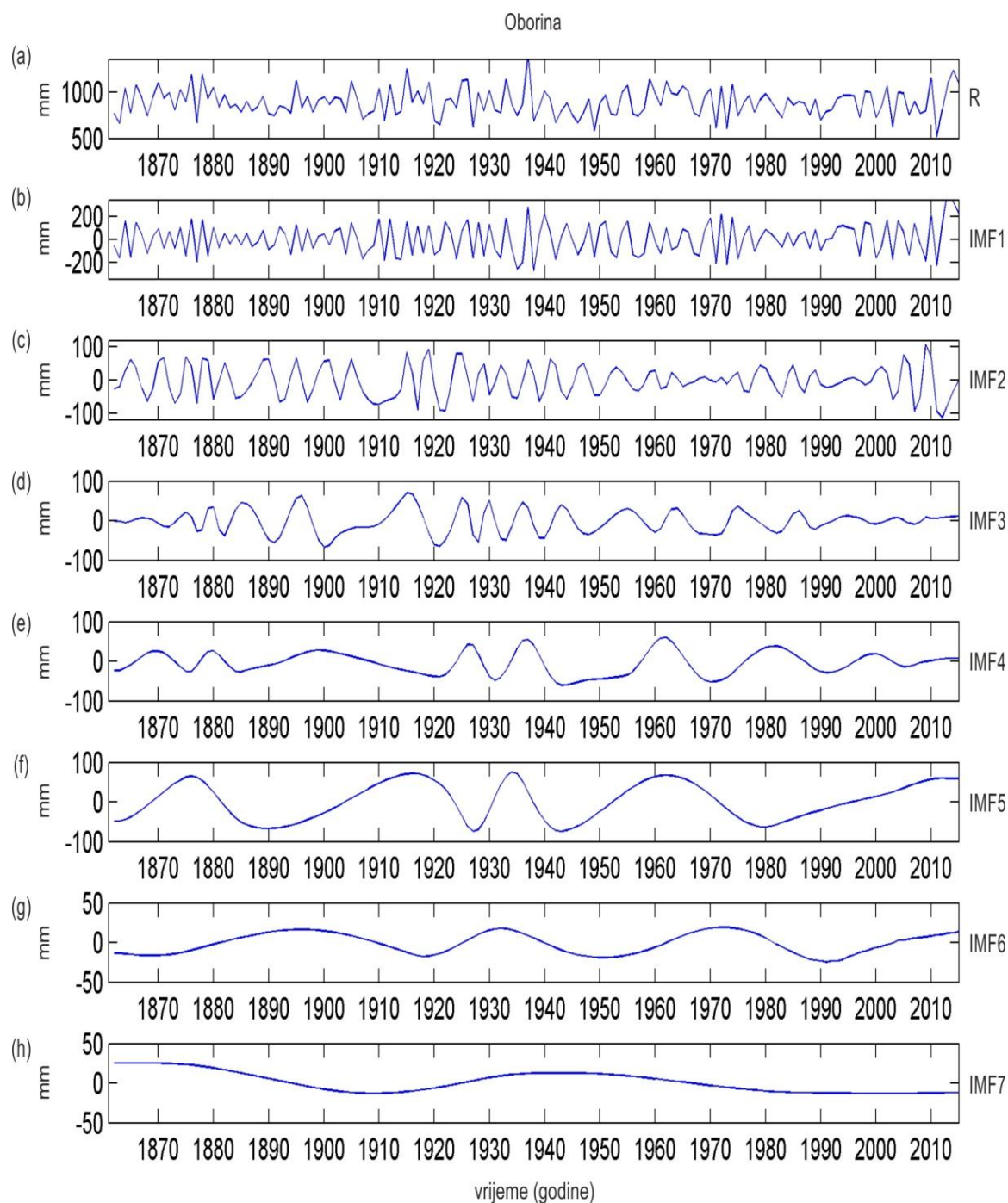
Slika 6. Isto kao slika 2, samo za niz godišnjih suma oborine.
