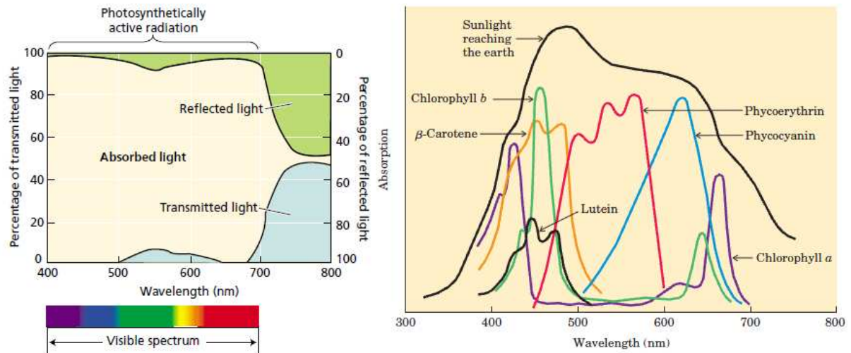
Slika 3. Apsorpcijski spekter lista (lijevo) i nekih fotopigmenata (desno) (prema Nelson i Cox, 2005).
