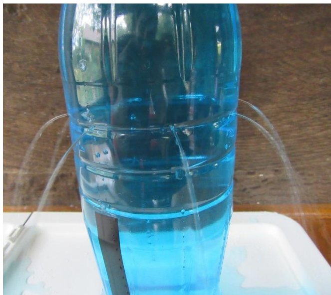
Slika 4.3. Plastična boca s rupicama na istoj visini.
