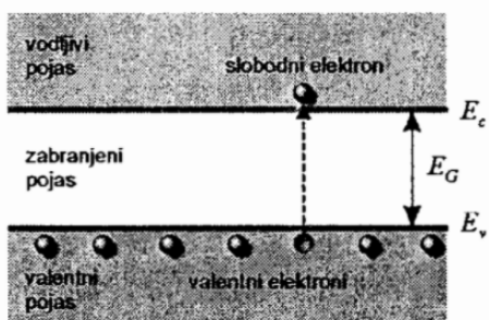
Slika 2.1: Prikaz energijskih vrpki poluvodiča. Naznačeni su rubovi valentne ( E_v ) i vodljive vrpce ( E_c ), kao i energijski procjep E_G . [1]
