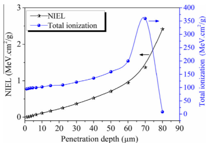
Slika 4.1: Prikaz izmjerenih vrijednosti ukupnog gubitka energije ionizacijom protona energije 2.55 MeV-a prilikom prolaska kroz silicijsku metu. Odsjekom krivuljom je prikazana i NIEL komponenta. Izvor: [13]
