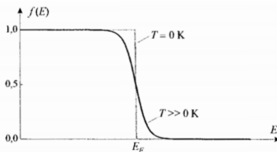
Slika 2.2: Fermi-Dirac funkcija vjerojatnosti. Na 0 K funkcija ima oštar rub (stepenica) na Fermij energiji E_F . Na višim temperaturama javlja se razmazanost raspodjele vjerojatnosti. [1]
