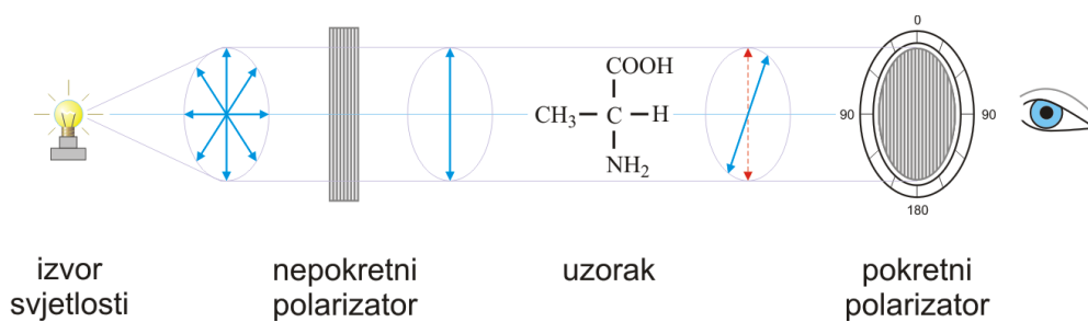
Slika 5. Zakretanje ravnine polarizirane svjetlosti kiralnog alanina. 5
