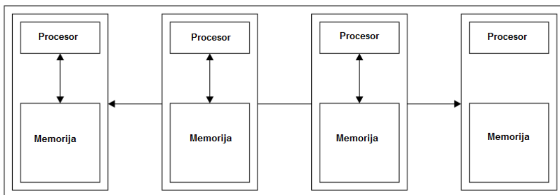
Slika 1.2: Distribuirani sustav
