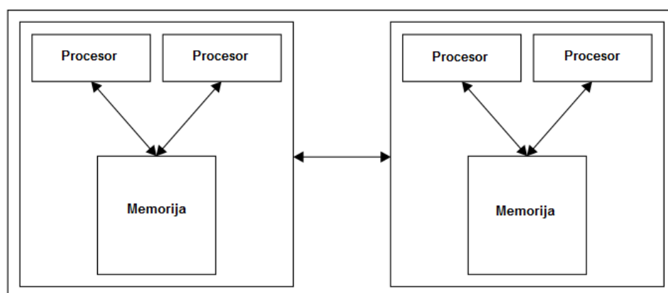
Slika 1.3: Hibridni sustav
