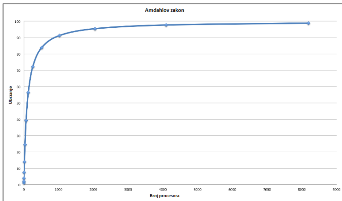
Slika 1.4: Predikcija Amdahlovog zakona [1]
