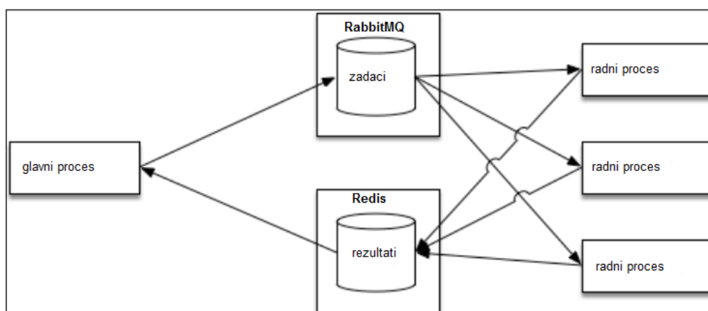
Slika 2.1: Celery arhitektura
