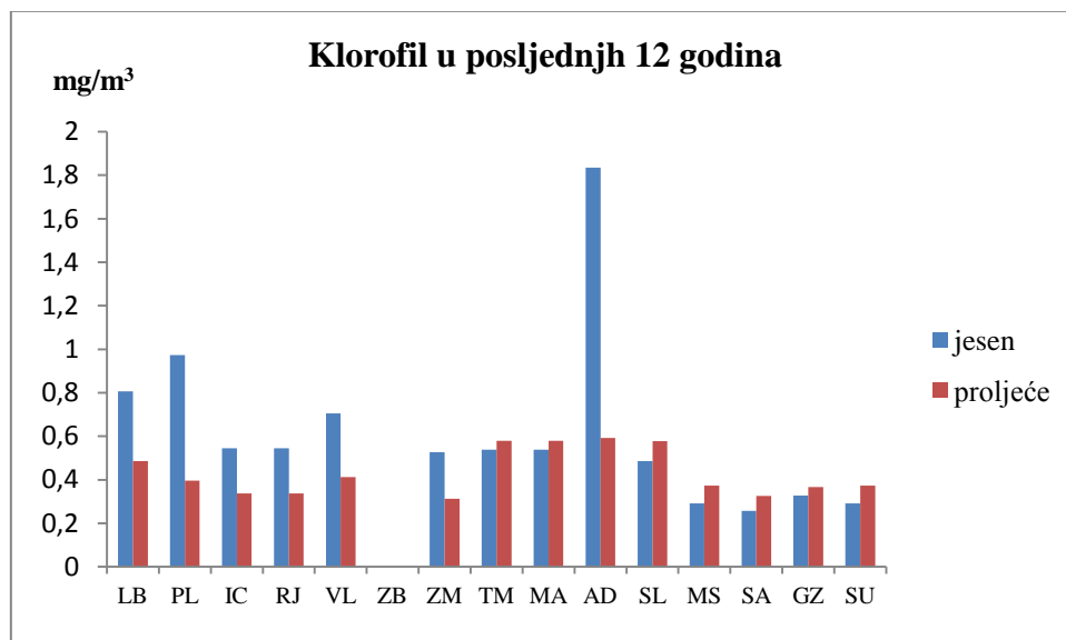
Slika 24. Vrijednosti klorofila u jesen i proljeće u posljednjih 12 godina preuzete s internetske baze podataka Ocean Color. (LB = Lijski zaljev, PL = Pula, IC = Ičići, RJ = Rijeka, VL = Viktor Lenac, ZB = Seline, ZM = Zadar Marina, MA = Marina, TM = Trogir Marina, AD = Adriavinil, SL = Split, MS = Mali Ston, SA = Mljet, GZ = Gruž).
