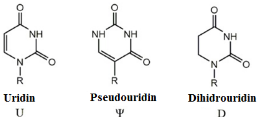
Slika 9 Strukturne formule uridina i njegovih modificiranih derivate - pseudouridina i dihidrouridina.
