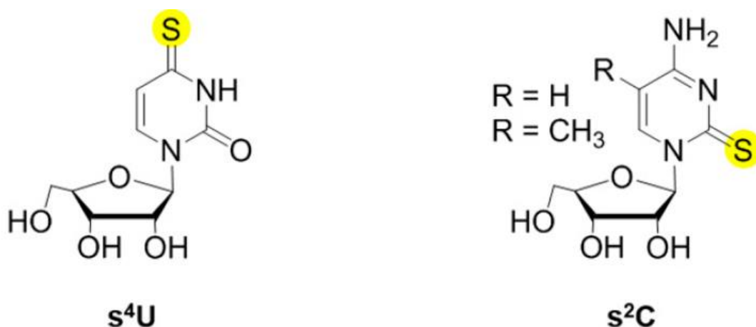
Slika 16 Strukturne formule najčešćih tionukleozida: 2-tiouridin i 2-tiocitozia.
