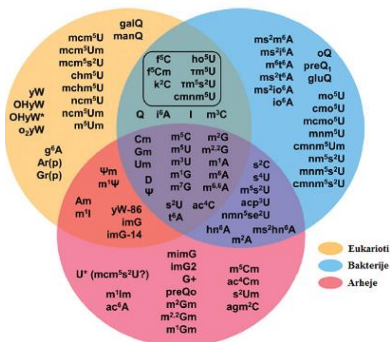
Slika 6 Vennov dijagram kemijskih modifikacija tRNA pronadenih kod barem jedne vrste eukariota, bakterija i arheja. Uokvirene modifikacije pripadaju molekulama tRNA organela. Značenje simbola i kratica modifikacija objašnjena je u nastavku. m n X – metilacija na poziciji nukleotida baze X; m n,n X – dimetilacija na poziciji nukleotida baze X; s n X – zamjena kisika sumporom na poziciji n nukleotida X; X m – 2'-O metilacija nukleotida X; D – dihidrouridin; Ψ – pseudouridin; ac 4 C – N-4 acetilcitidin; i 6 A – izopenteniladenozin; t 6 A – N-6 treoniladenozin; g 6 A – N-6 glicinilkarbamoidadenozin; io 6 A – N-6 (cis-hidroksipentenil)adenozin; hn 6 A – N-6 hidroksinorvalilkarbamoidadenozin; ac 6 A – N-6 acetidiladenozin; Xr(p) – 2'-O ribozilfosfatni derivat nukleotida X; f 5 C – formilcitozin; k 2 C – lizidin; agm 2 C – agmatidin; acp 3 U – 3-(3-amino-3-karboksipropil)uridin; mcm 5 U, C-5 metoksikarbonilmetil uridin; mnm 5 U – C-5 karbamoidmetil uridin; chm 5 U – C-5 karboksihidroksimetil uridin; ho 5 U – C-5 hidroksiuridin; mo 5 U – C-5 metoksiuridin; cmo 5 U – uridin 5-oksiacetilna kiselina; mcmo 5 U – uridin 6-oksiacetilna kiselina metilester; mnm 5 U – C-5 metilaminometiluridin; cmnm 5 U – C-5 karboksimetilaminometiluridin; nm 5 U – C-5 aminometiluridin; Q – kveozin (i srodne 7-deaza vrste – oQ, preQ 1 , preQ 0 , gluQ, galQ, manQ); G+ – arheozin; yW – vibutozin (i srodne OHyW, OHyW*, o 2 yW i yW vrste); imG – viozin (i srodne imG-14, mimG i imG2 vrste).
