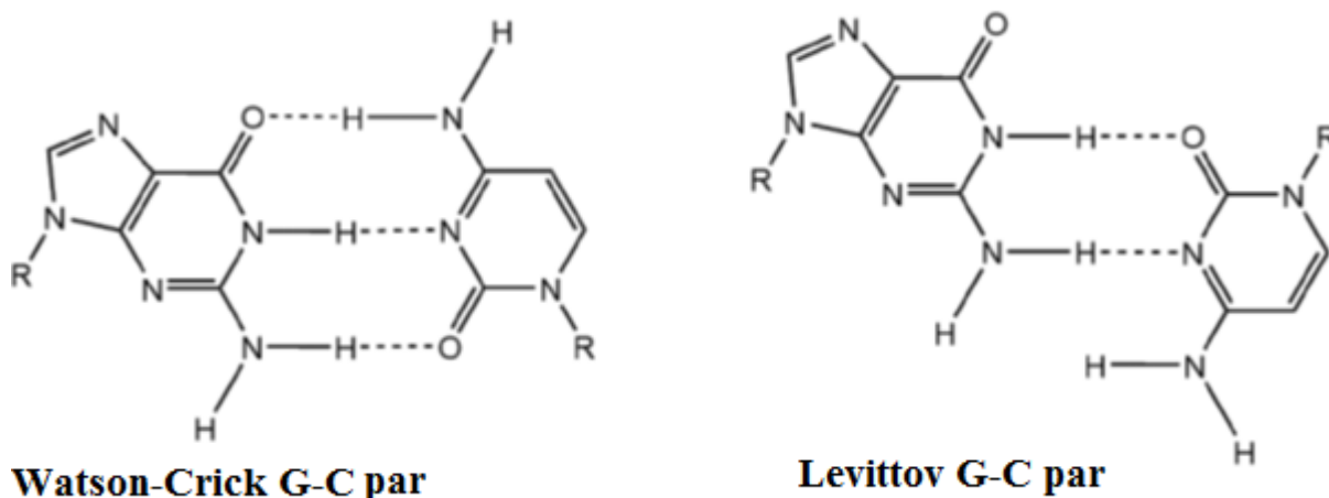
Slika 10 Razlika u sparivanju Watson–Crick parova i Levitt baznog para.
