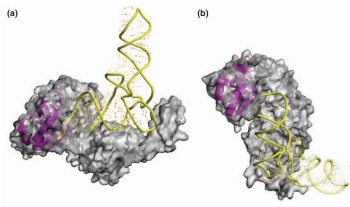
Slika 5 Kristalne strukture kompleksa tRNA vezane za nukleotidil-transferazu a) skupine I, b) skupine II. (Y. Xiong, T. A. Steitz, Cur. Op. in Struct. Biol. , 16 (2006) 12–17)
