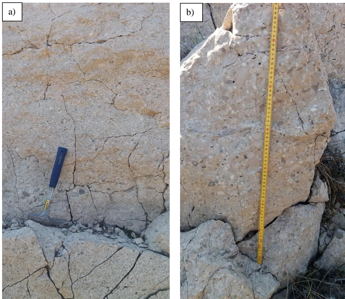
Slika 11. Facijesna asocijacija D. (a) Klastpotporni, srednje sortirani konglomerati (Facijes D1). (b) Matrikspotporni, loše sortirani konglomerati (Facijes D2).
