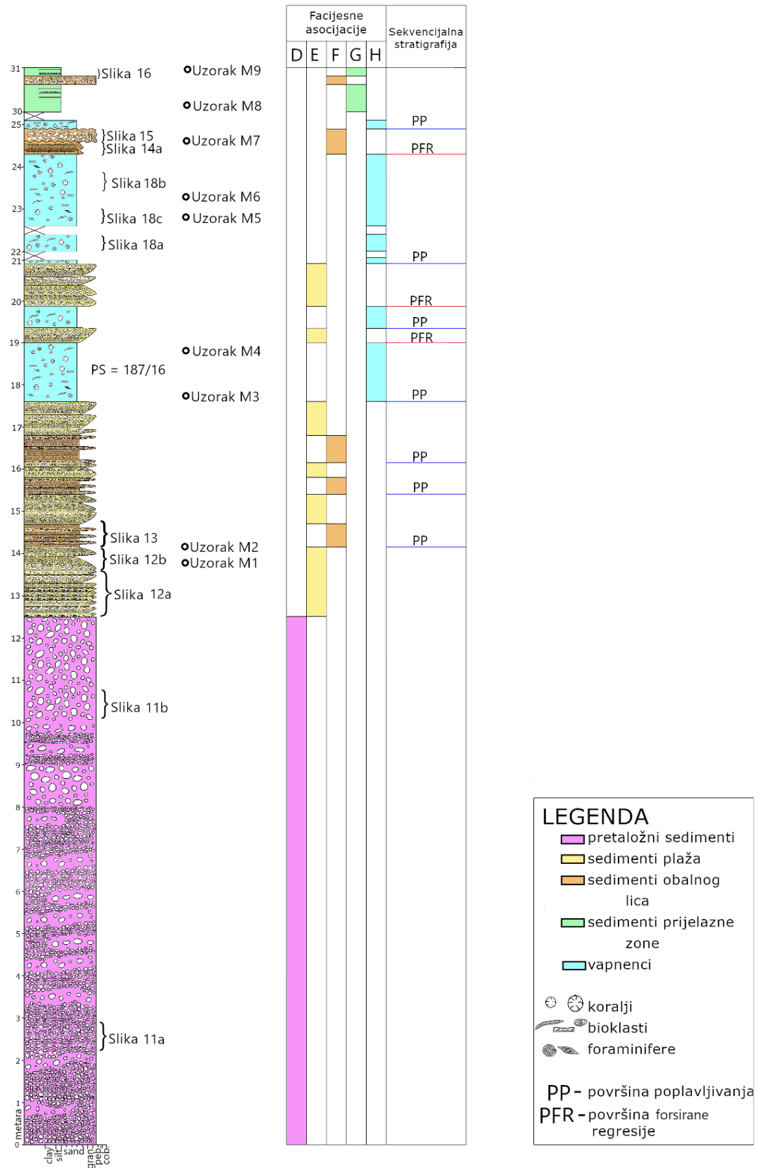
Slika 22. Prikaz detaljnog sedimentološkog stupa „STUP MASLENICA 2“ s izdvojenim facijesnim asocijacijama, površinama poplavljivanja i forsirane regresije, legendom te s naznačenim položajem sloja, mjestom uzorkovanja i snimanja fotografija.
