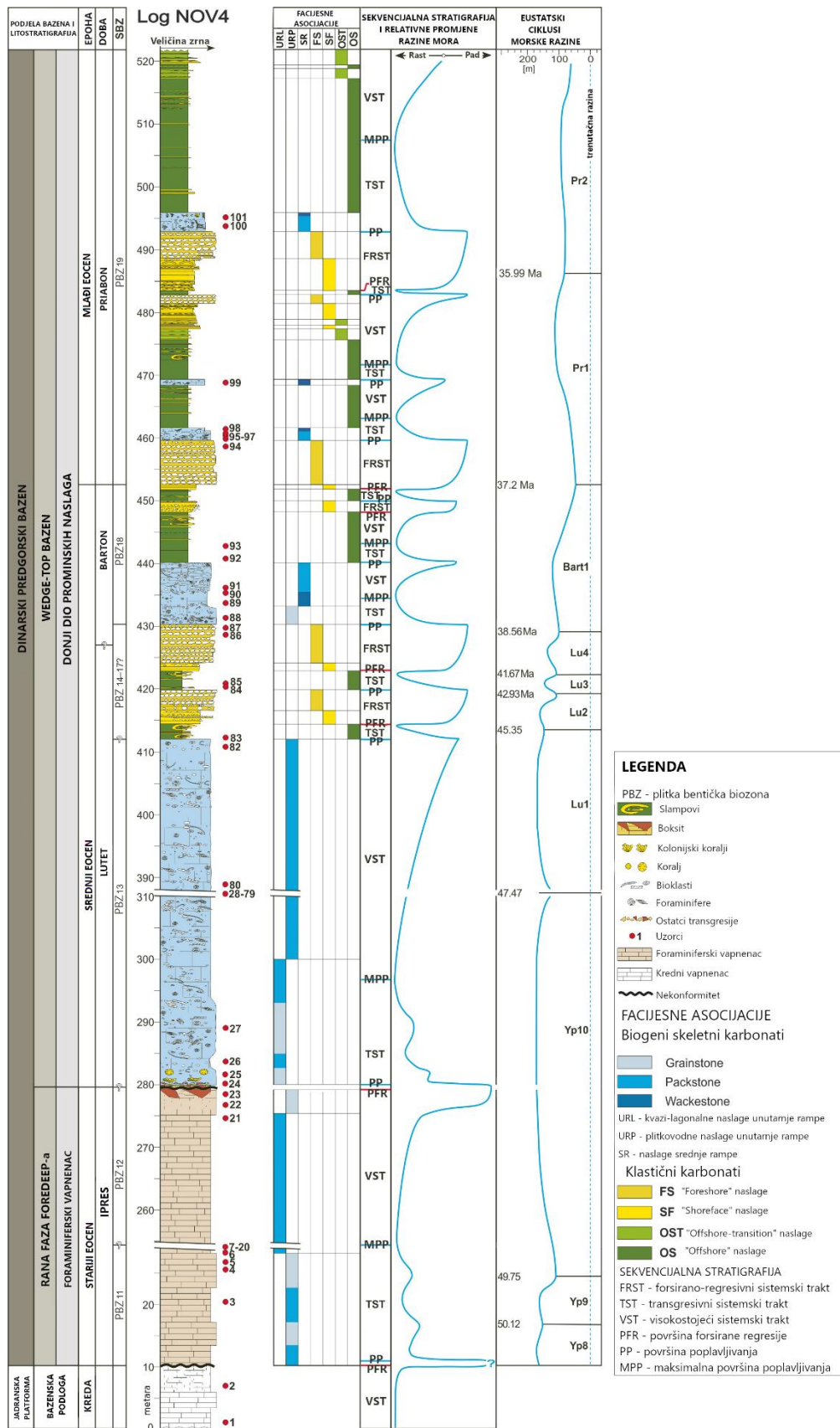
Slika 24. Prikaz detaljnog sedimentološkog stupa „Log NOV4“ s izdvojenim facijesnim asocijacijama, legendom te s naznačenim mjestom uzorkovanja (preuzeto i modificirano prema Čosović et al., 2018).
