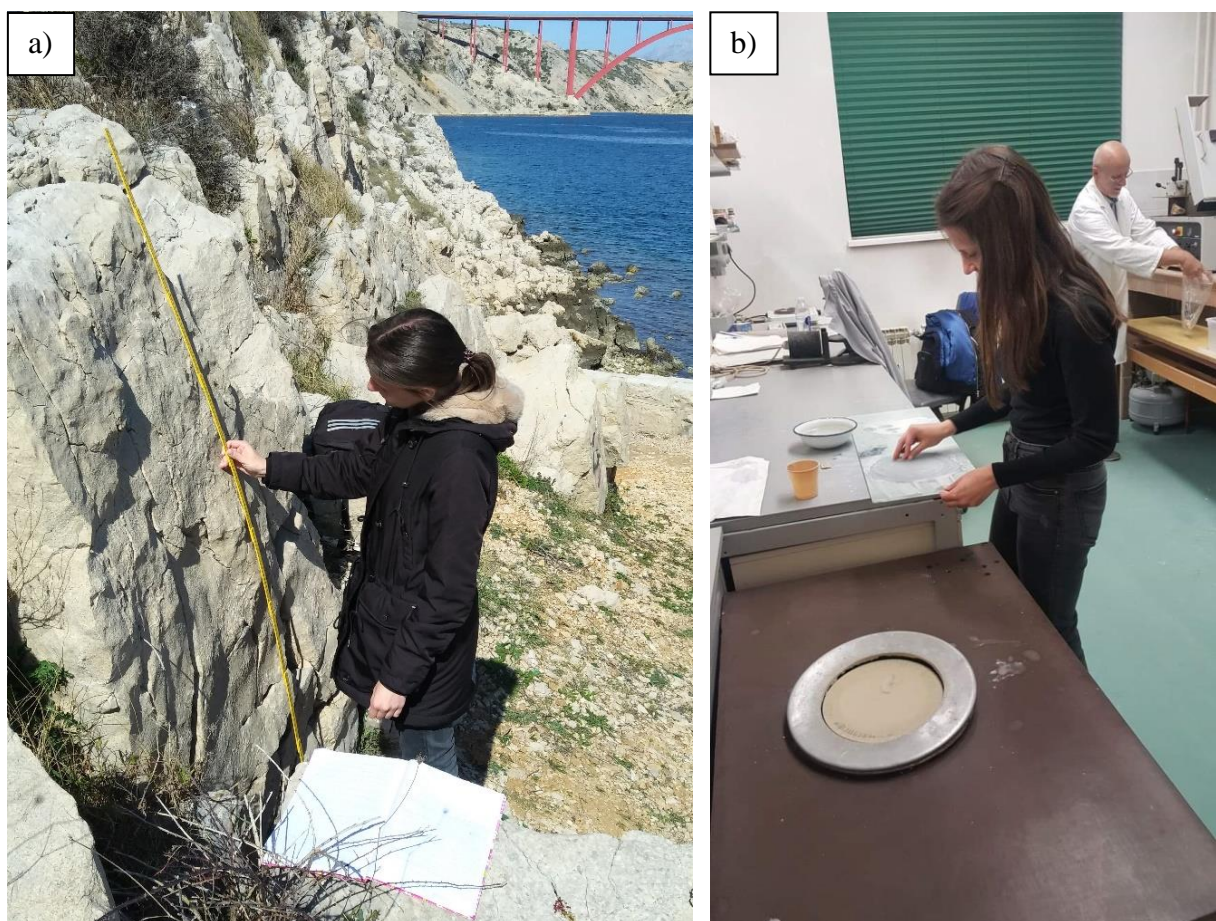
Slika 7. (a) Snimanje sedimentološkog stupa na izdanku. (b) Izrada izbrusaka.
