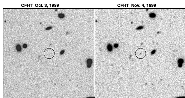
Slika 2. Supernova SN 1999fv (nazvana “Dudley DoRight”, prema popularnom junaku iz stripova) jedna je od najudaljenijih otkrivenih supernova. Nalazila se na udaljenosti od 8 milijardi svjetlosnih godina ( z = 1.23 ) i udaljavala se od nas brzinom od 80% brzine svjetlosti.
