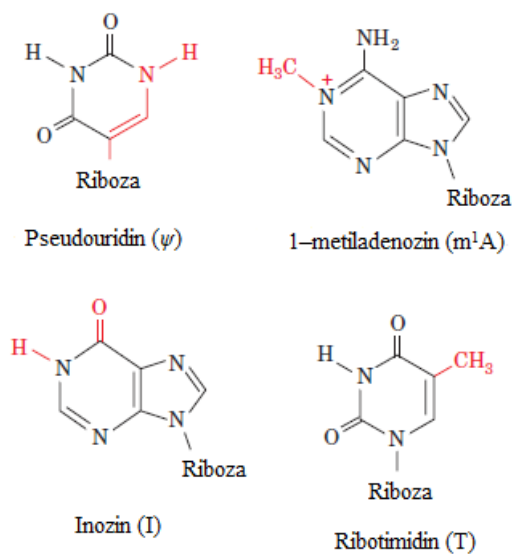
Slika 2.2. Kemijske strukture nekih od modificiranih nukleotida koji se mogu nalaziti u molekulama tRNA. Slika je preuzeta i prilagođena prema ref. 20.
