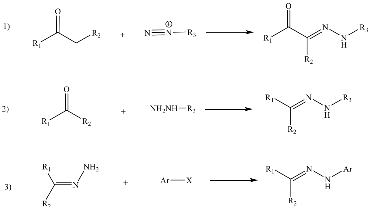
Shema 1. Sinteza hidrazona 1) Japp-Klingenmanova reakcija, 2) kondenzacija aldehida / ketona s hidrazidom, 3) reakcija nesupstituiranog hidrazona s aril-halogenidom
