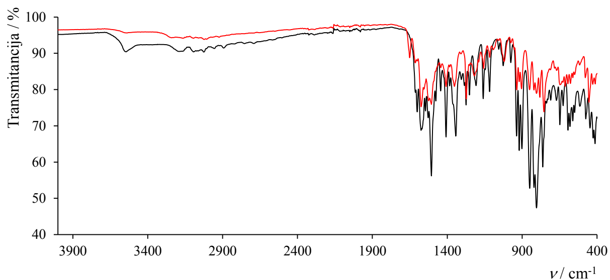
Slika D31. IR spektar kompleksnog spoja [CuMoO 2 (L)(H 2 O) 2 ]
