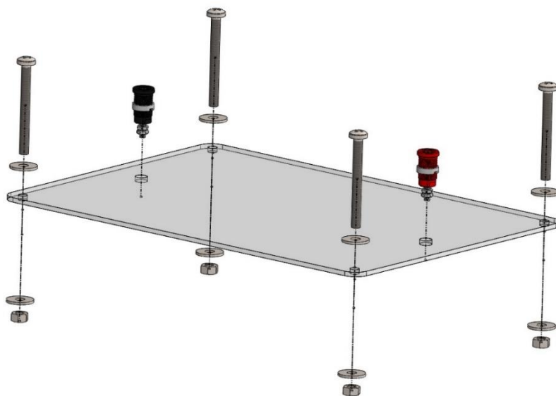
Slika 16 Način sklapanja stalka
