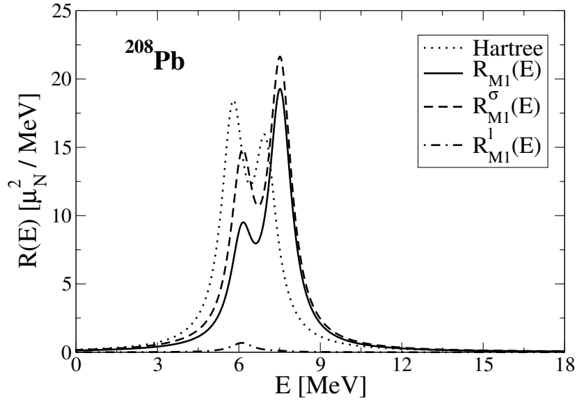
Slika 3.2: Isto kao na slici 3.1, ali sa R_{M1}(E) -ukupnom, R_{M1}^σ(E) -spinskom i R_{M1}^l(E) -orbitalnom funkcijom odziva. Neperturbirani Hartree odziv je također prikazan.
