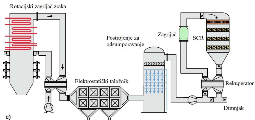
Slika 6-1. Mogući položaji SCR uređaja kod uređaja za loženje (APO d.o.o. i EKONERG d.o.o., 2012.c)
