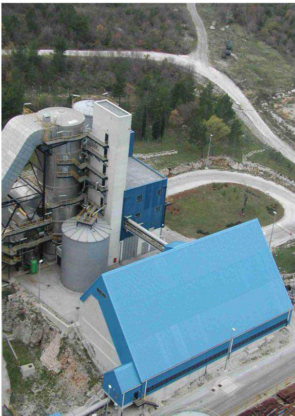
Slika 4-11. Postrojenje za odsumporavanje dimnih plinova (DeSO x ) TEP 2 (Vukelić, 2013.)
