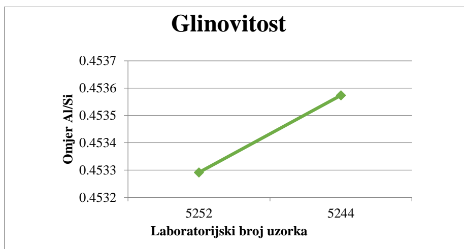
Slika 6-17. Prikaz geokemijskog omjera Al/Si koji ukazuju prvenstveno na hidrolizu
