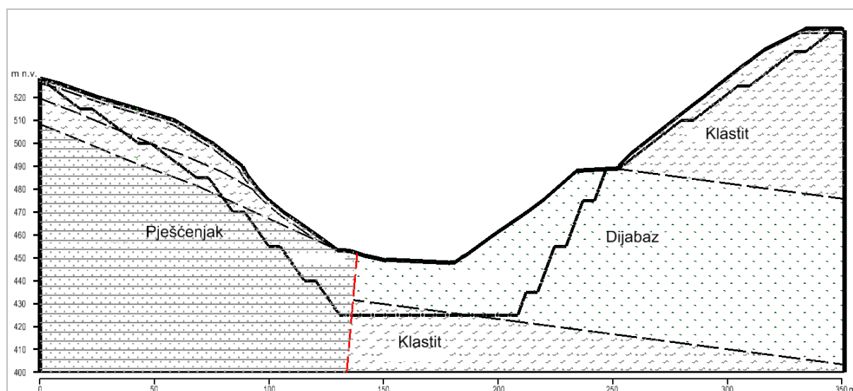
Slika 1.4 Karakteristični profil istočnog dijela kopa
