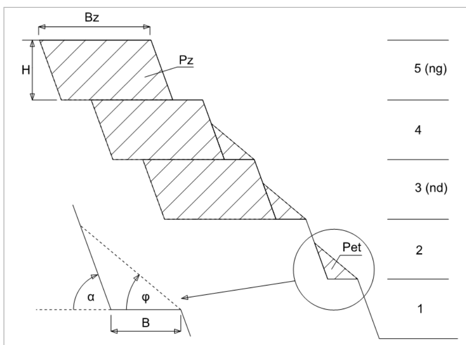
Slika 2.10 Shema i princip izračuna obujma prebacivanja
