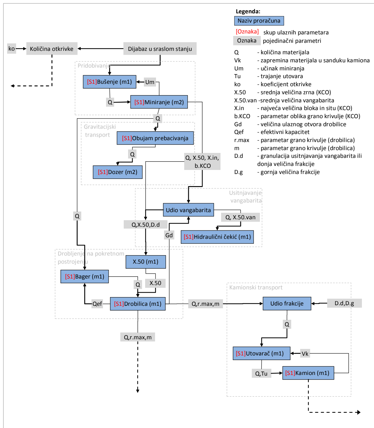
Slika 4.1 Isječak računske sheme
