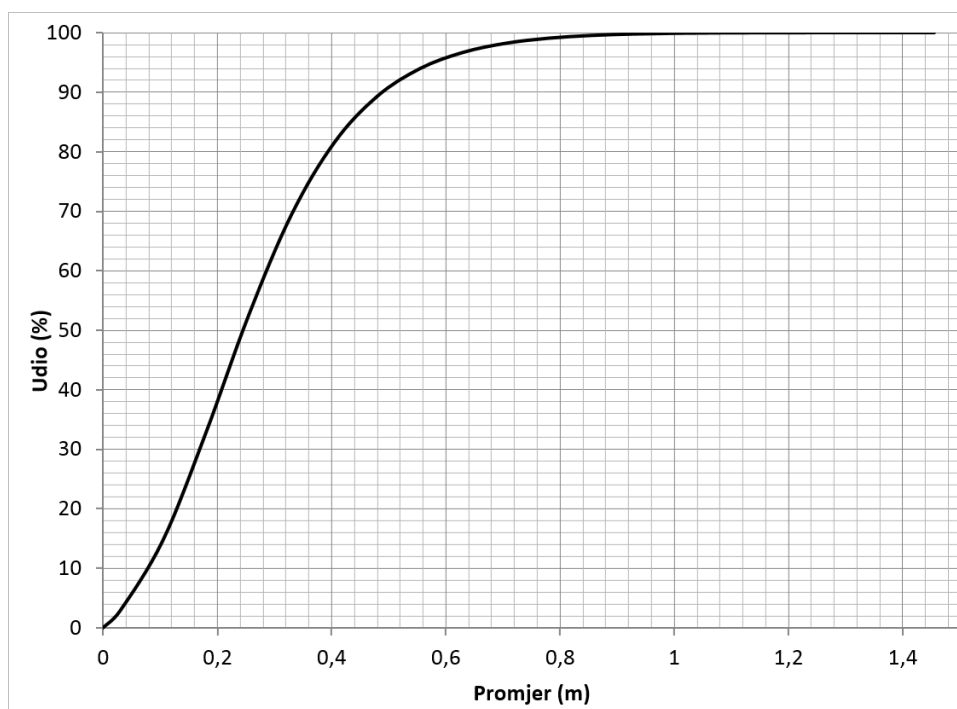
Slika 3.2 Fragmentacijska krivulja KCO modela
