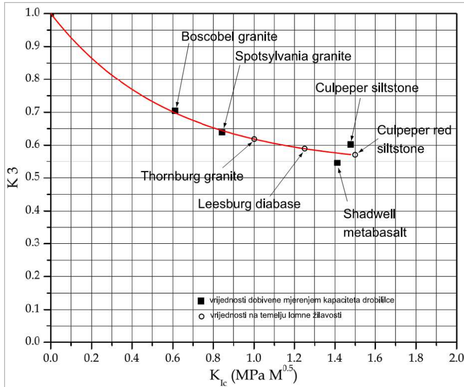
Slika 2.14 Zavisnost parametra K_3 o lomnoj žilavosti (modificirano prema Donovan, 2003)
