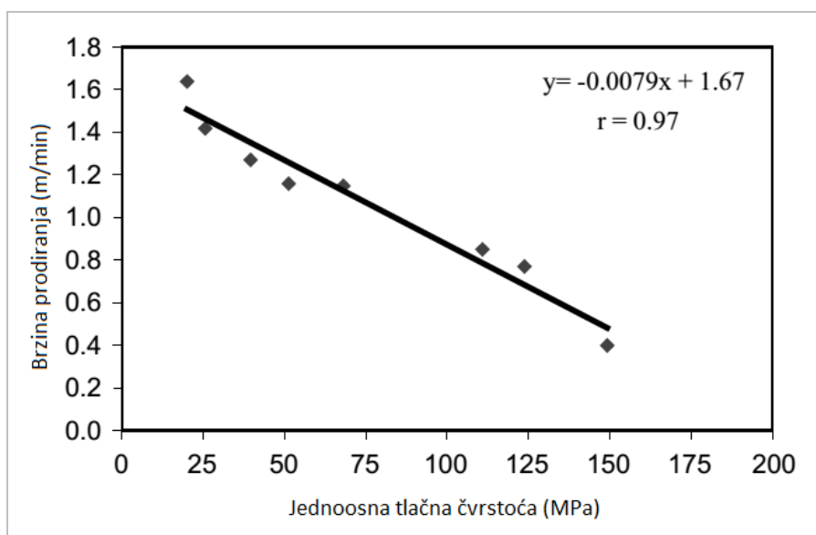
Slika 2.6 Korelacija brzine čistog bušenja i jednoosne tlačne čvrstoće (Kaharman et.al,2003)
