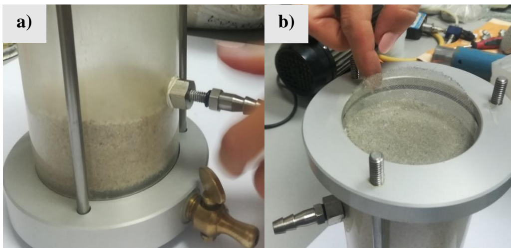
a) zavrtnjanje manometarske spojnice do konačnog položaja b) postavljanje filtarske mrežice na vrh uzorka
