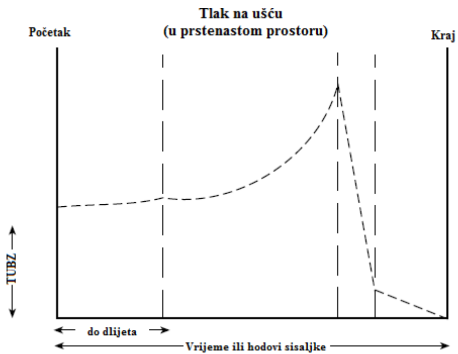
Slika 4-5. Razvoj tlakova na ušču tijekom provođenja inženjerske metode (Aberdeen Drilling School, 2002)
