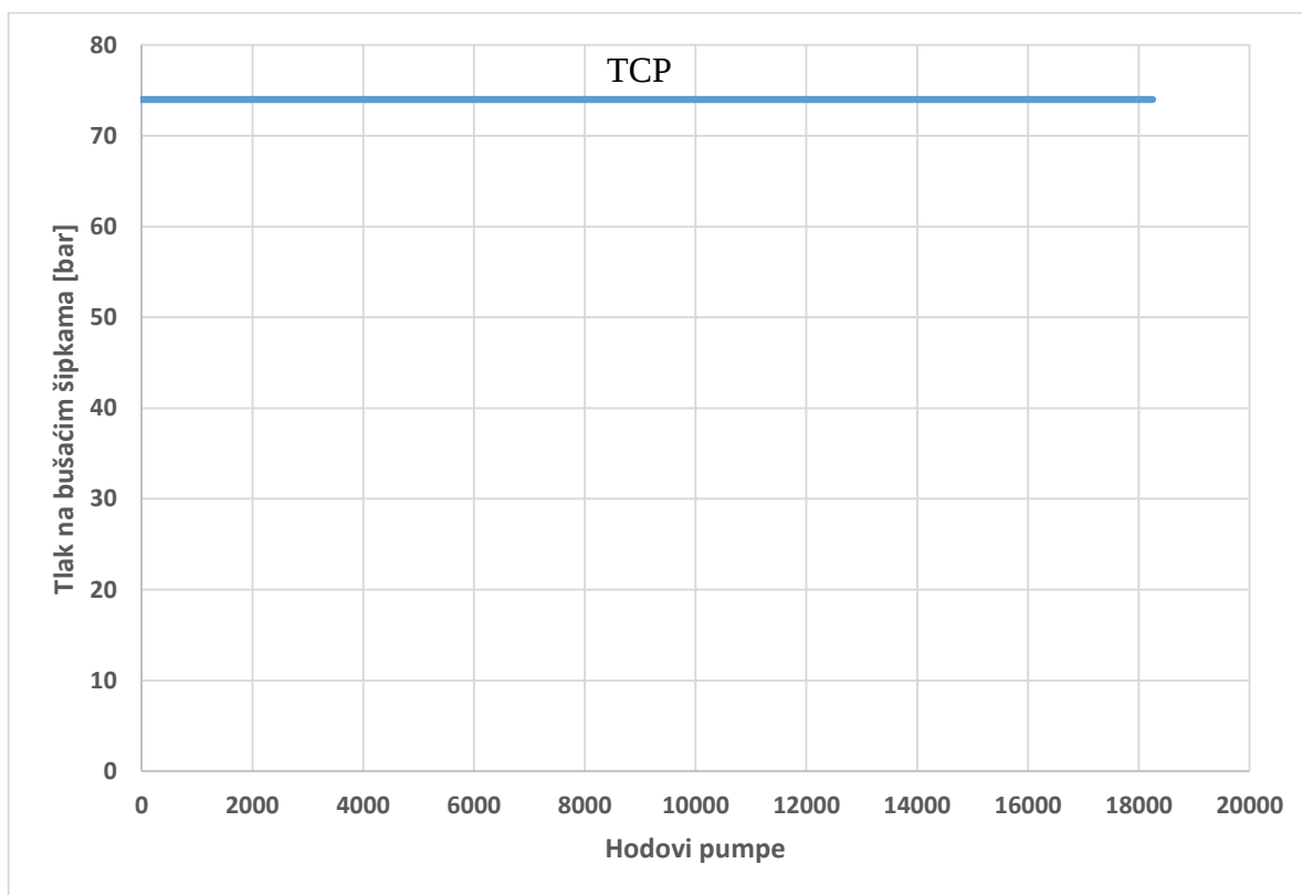
Slika 5-3. Tlak na bušačim šipkama tijekom prve cirkulacije bušaće metode
