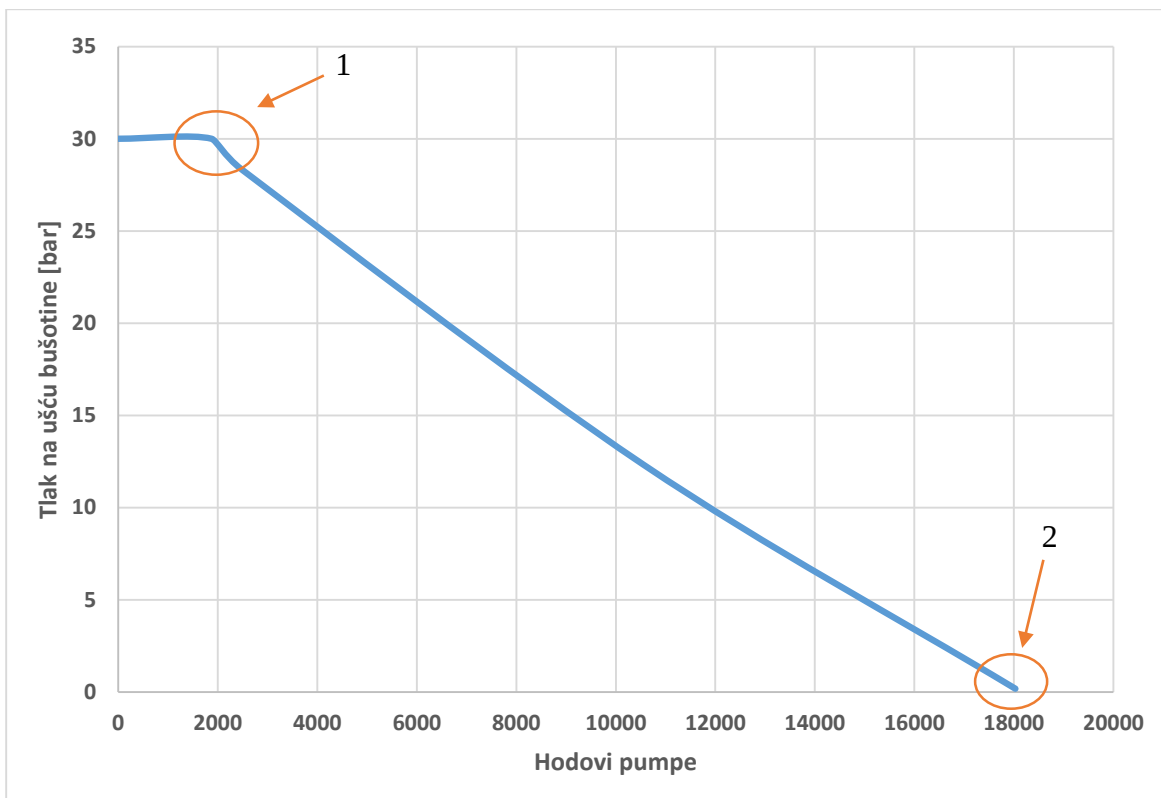
Slika 5-6. Tlak na ušću bušotine tijekom druge cirkulacije bušaće metode
