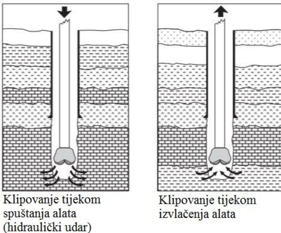
Slika 2-1. Prikaz klipnog efekta (Aberdeen Drilling Schools, 2002).
