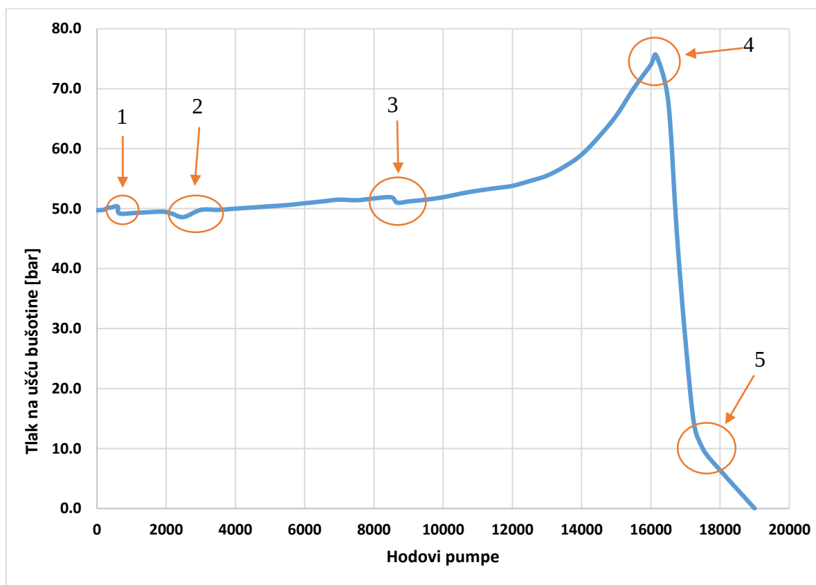
Slika 5-8. Tlak na ušću bušotine tijekom inženjerske metode.
