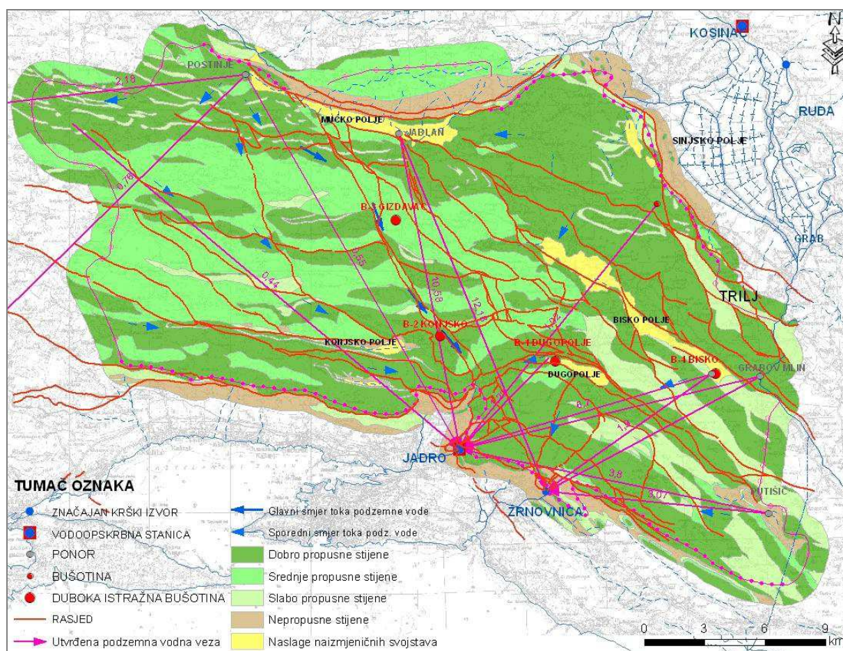
Slika 5.1. Shematska hidrogeološka karta sliva
