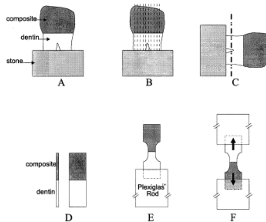
Slika 26. Microtensile bond strength test (preuzeto iz 103).
