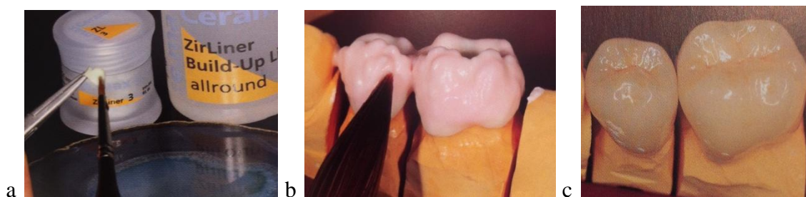
Slika 19. a) nanošenje veznog sredstva b) nanošenje obložne keramike c) gotovi rad (Prikaz slučaja preuzet iz 100).
