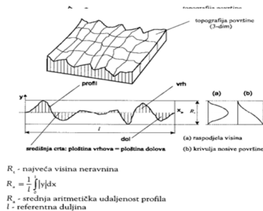
Slika 20. Topografija i karakteristike hrapavosti površine (preuzeto iz 53).
