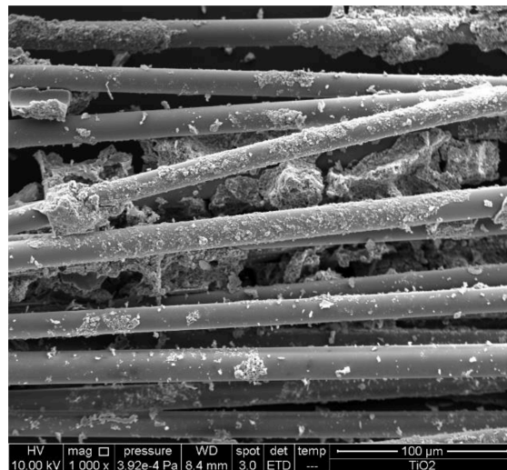
Slika 31. SEM prikaz staklene mrežice s \text{TiO}_2 koji je vezan na mrežicu sol – gel metodom.
