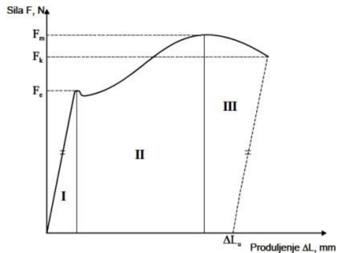
Slika 7. Dijagram sila-produljenje [4]
