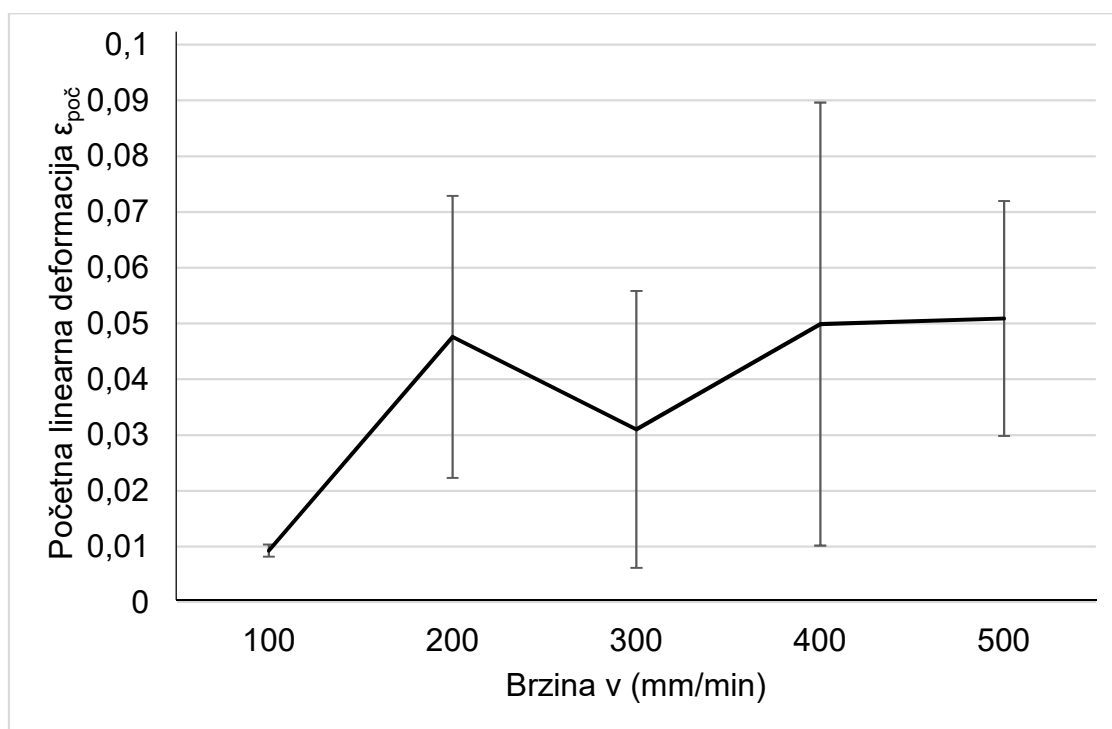
Slika 14. Dijagram odnosa srednjih vrijednosti početne linearne deformacije i brzine
