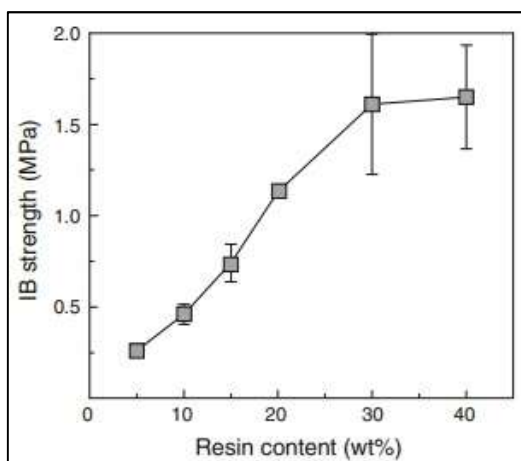
Slika 7. Utjecaj udjela adheziva na vlačnu čvrstoću (Izvor: Umemura i dr. 2013)
