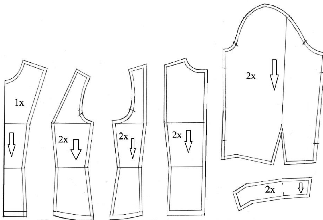
Sl.52. Dodavanje šavnih dodataka
