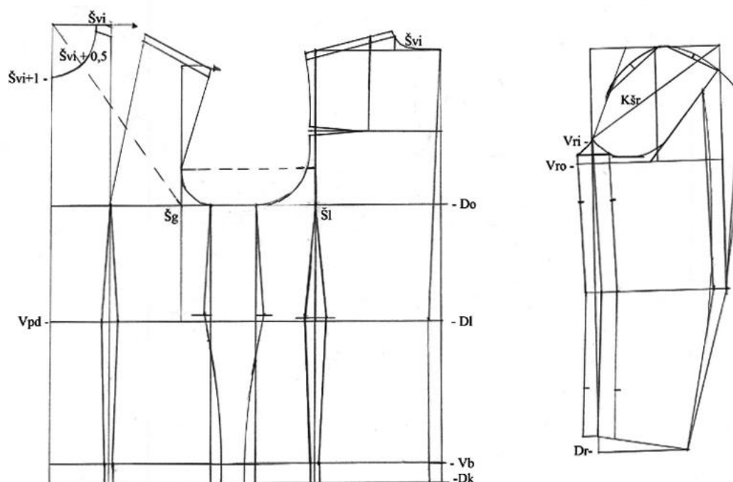
Sl.45. Temeljna konstrukcija jakne
