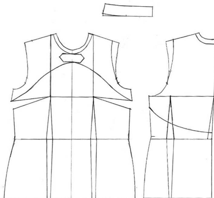
Sl. 48. Modeliranje Jakne
