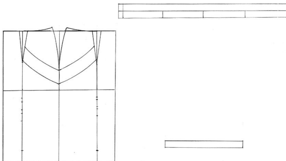
Sl.53. Modeliranje suknje
