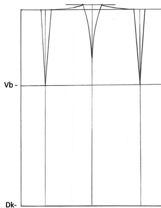
Sl.47. Temeljna konstrukcija suknje
