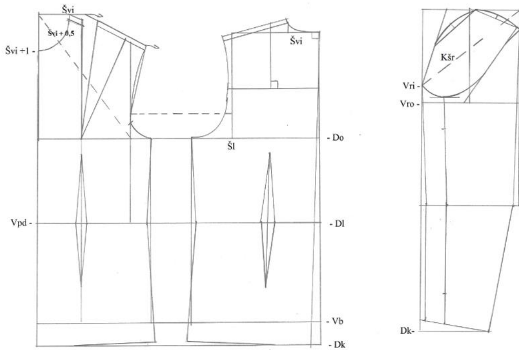
Sl.46. Temeljna konstrukcija bluže
