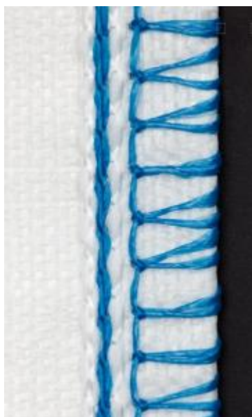
Sl. 1. Kombinacija šivaćih uboda u šivanom šavu (401.502)
